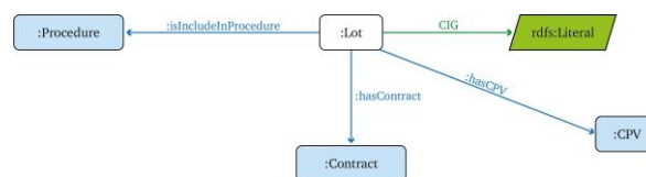
Figura 3.4: La classe “Lotto” e le sue relazioni
