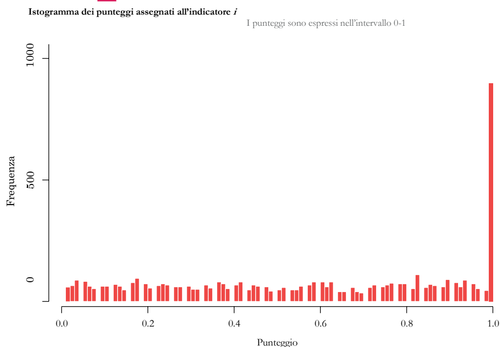
Figura 4.7: Istogramma dei punteggi indicatore I_{oepr2}
